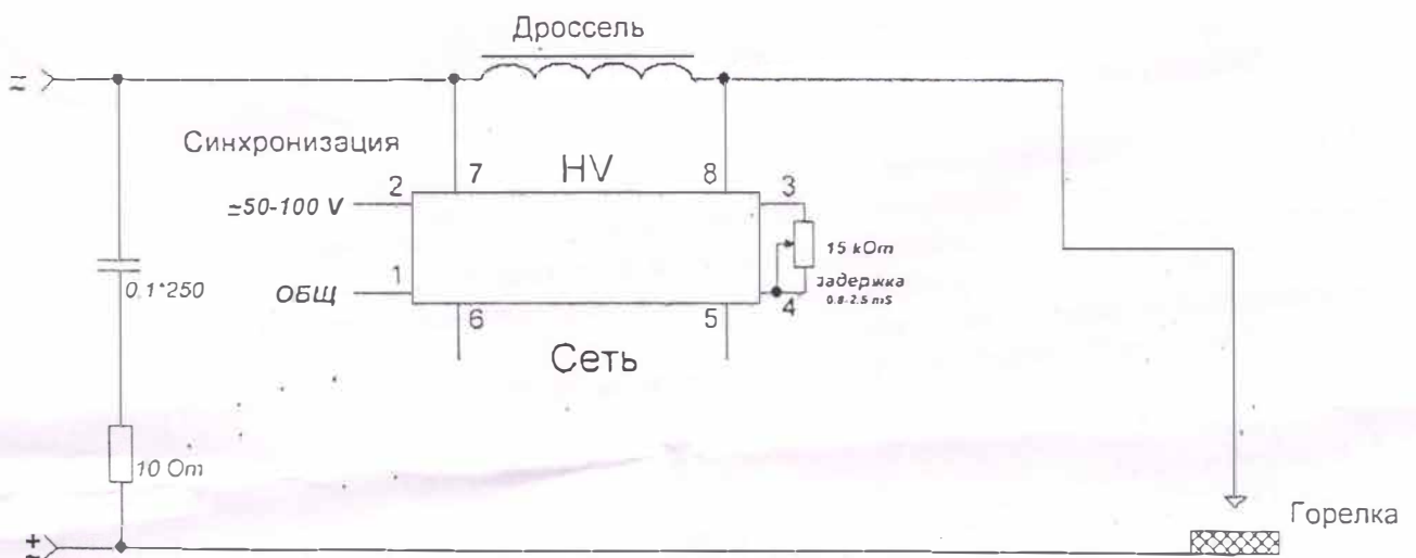
Рис 1 . Схема подключения.
